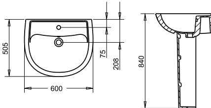
ALİZE (60 cm Lavabo + Kolon Ayak)
