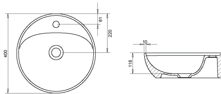
TOLEDOMİX (Batarya Delikli Çanak Lavabo)
