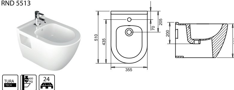
RONDO ASMA BİDE / Yandan Montaj RND 5513
