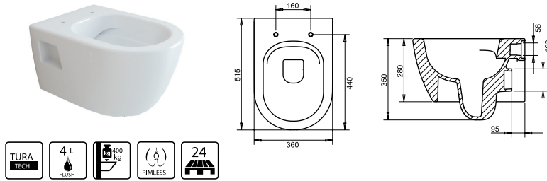
RONDO KANALLI ASMA KLOZET / Yandan Montaj RND 5508
