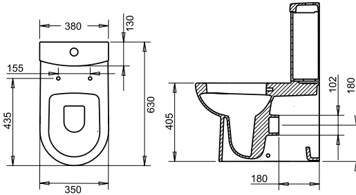
OMEGA DUVARA DAYALI KLOZET+SLIM REZERVUAR OMG 1303+1704
