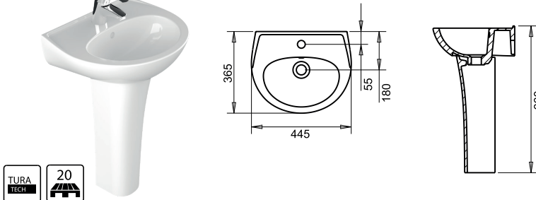
ÇOCUK KISA KOLON AYAK LAVABO 5003 + 5019
