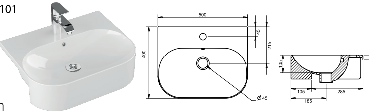
NEF LAVABO 40 X 50 cm NF 1101
