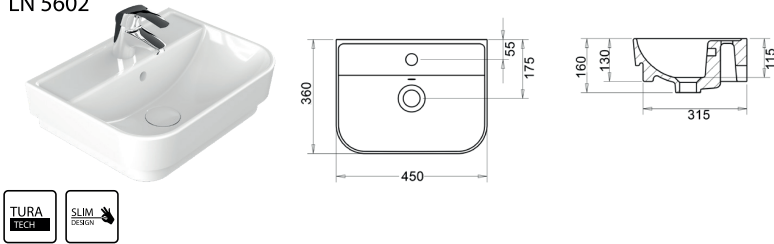
LUNA SLİM LAVABO 45 cm LN 5602
