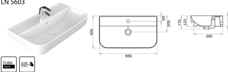
LUNA SLİM 65 cm LN 5603
